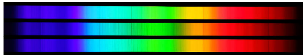
Lo spettro solare
